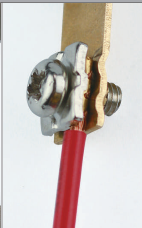
Serrage de la borne
