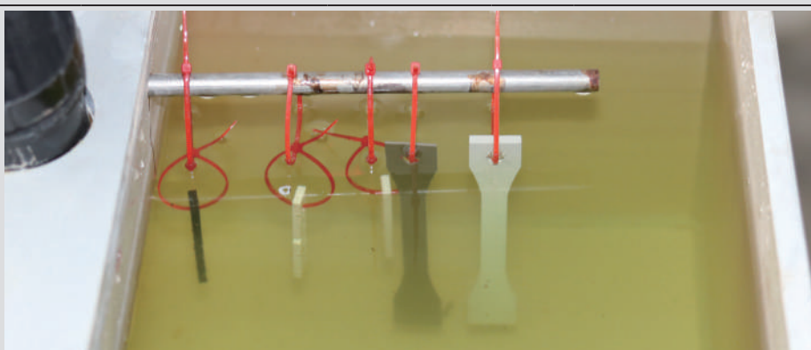
Position des spécimens dans le bain
