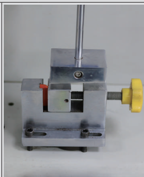
Eprouvette après essai Charpy
