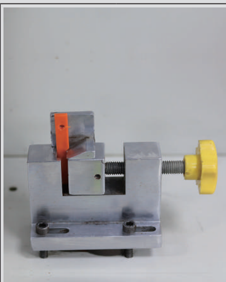
Eprouvette avant essai Charpy
