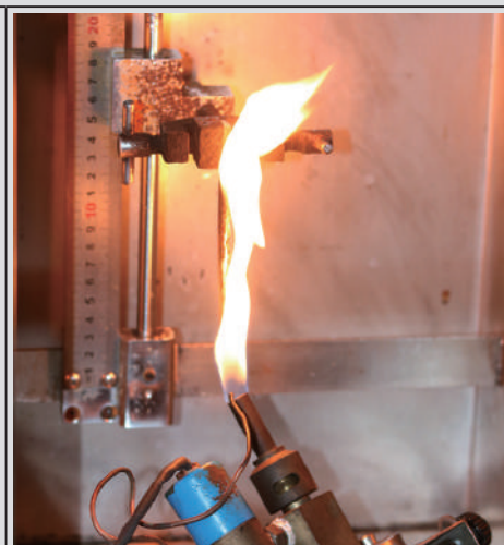
Eprouvette durant l'essai UL94 VO
